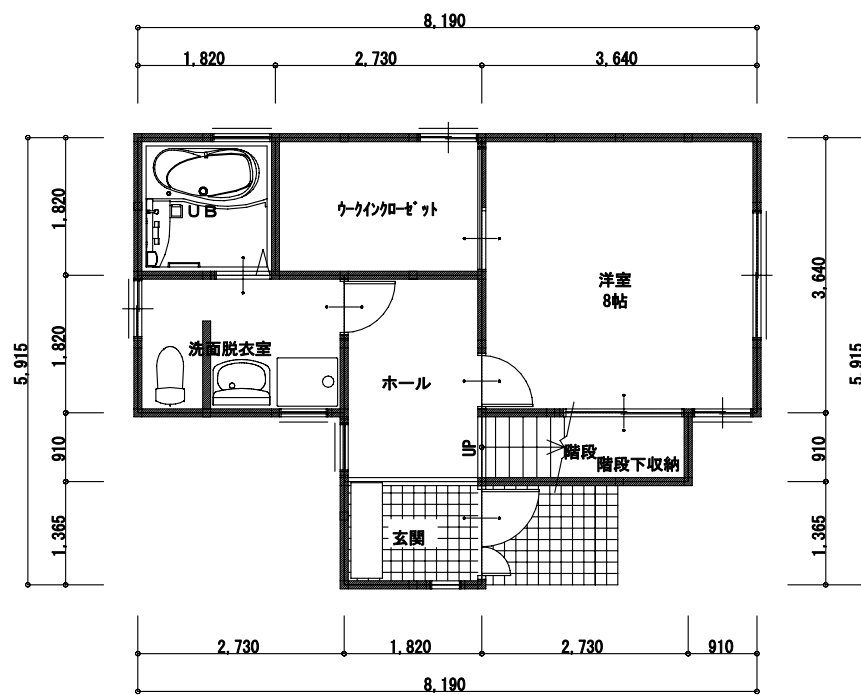
1階平面図
