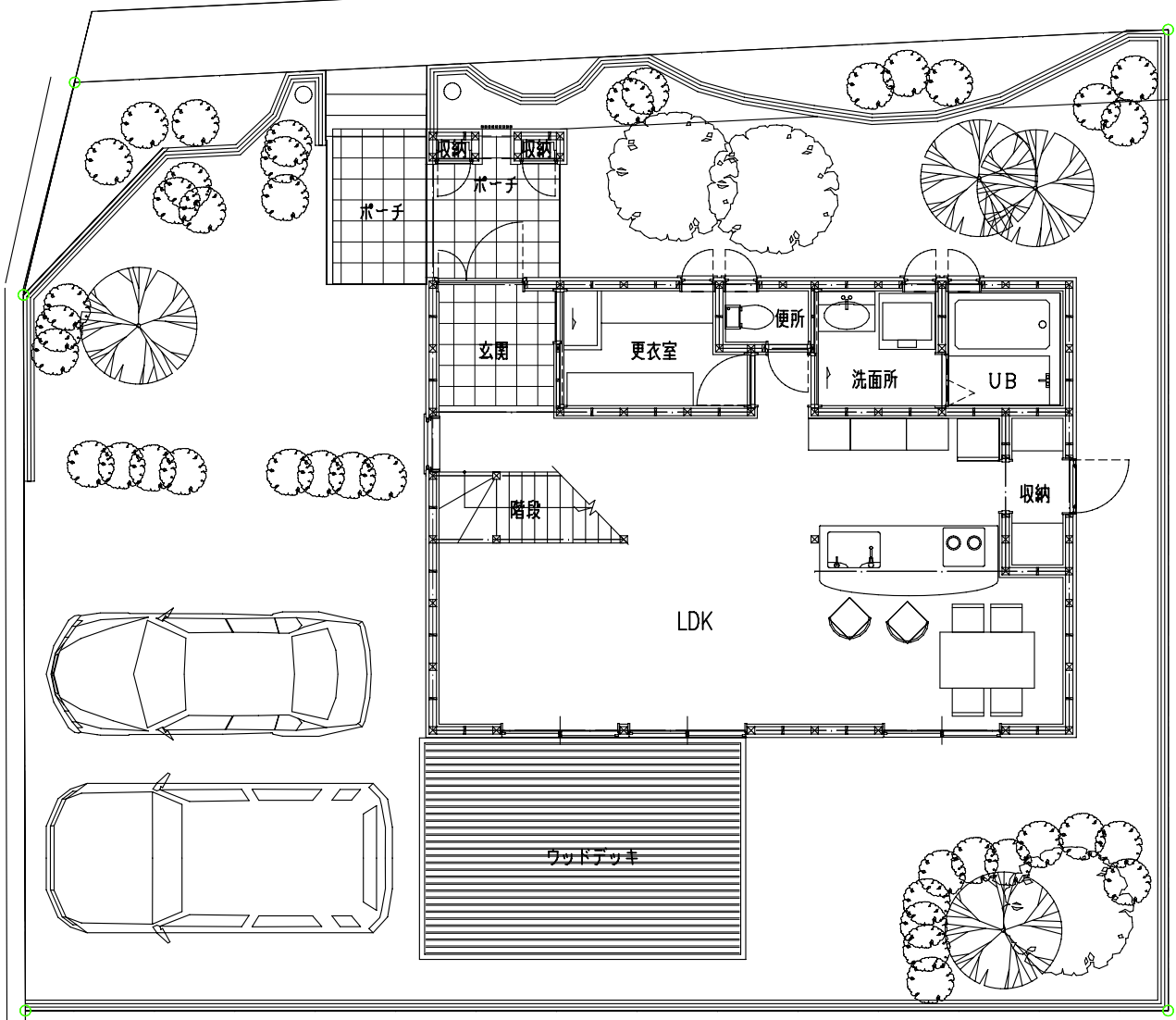
外構図 1:100
