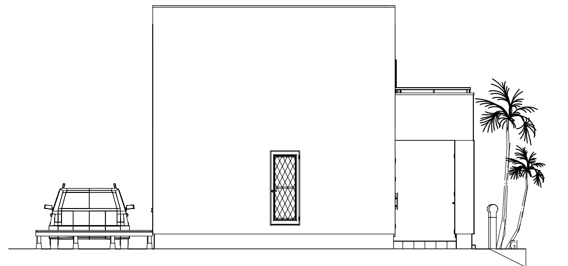
東立面図 1:100
