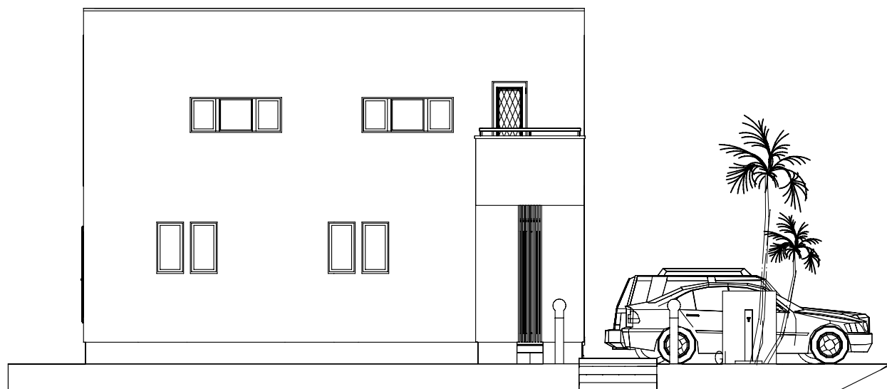
北立面図 1:100
