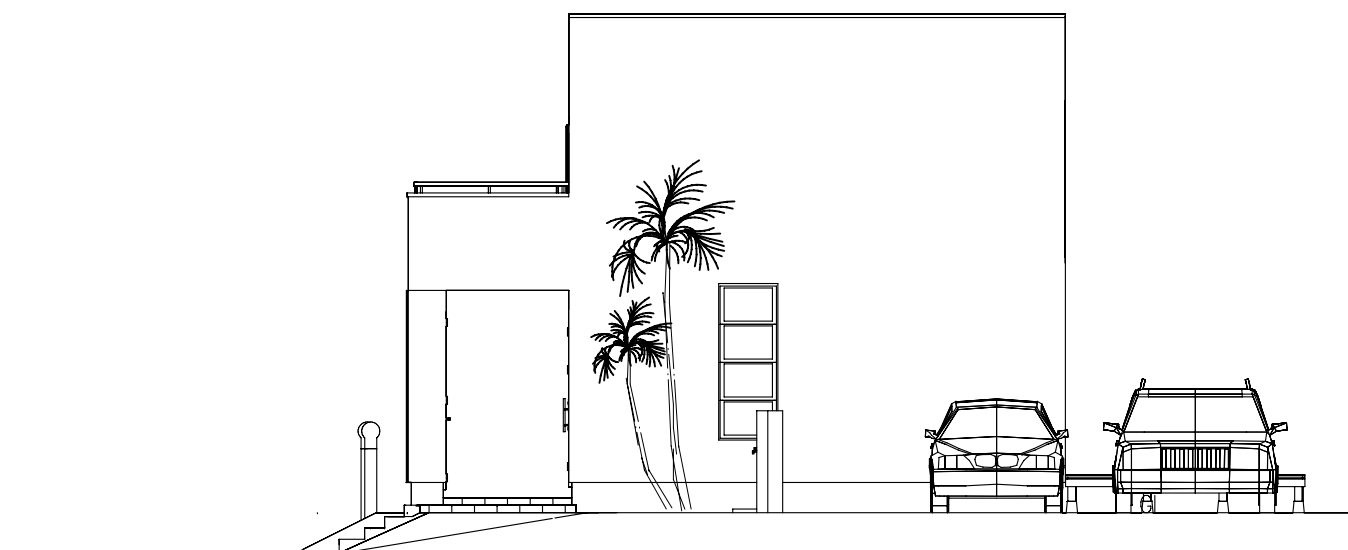
西立面図 1:100
